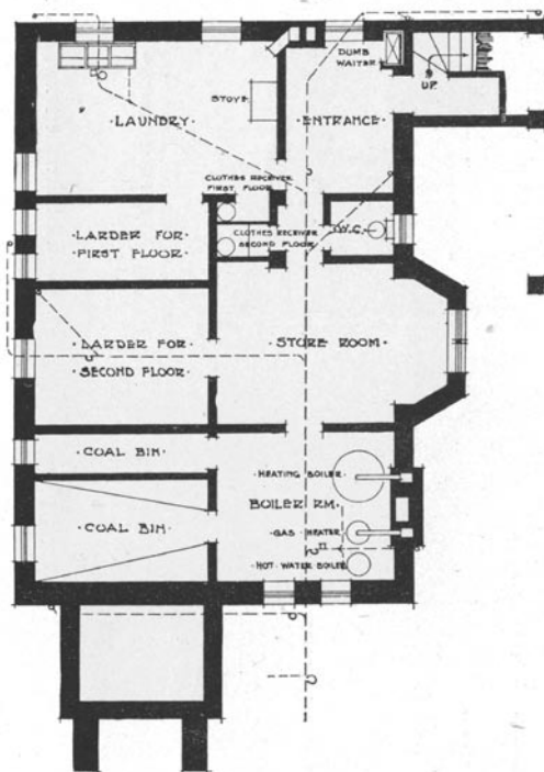
· BASEMENT · PLAN ·
